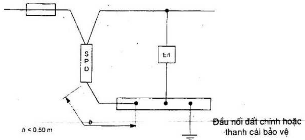
Hình 53E - Ví dụ về lắp đặt SPD tại hoặc gần điểm bắt đầu của hệ thống lắp đặt
