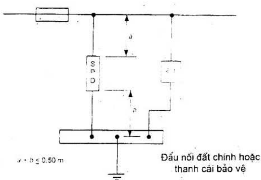
Hình 53D - Ví dụ về lắp đặt SPD tại hoặc gần điểm bắt đầu của hệ thống lắp đặt
